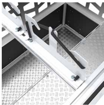
Gerätehalterungen
