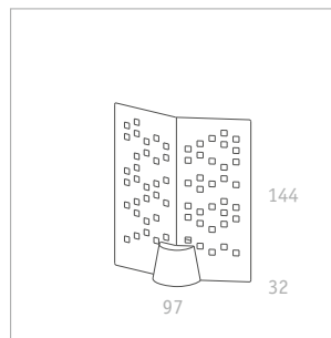
Separo Solo 1200 Weight 42,5 kg
